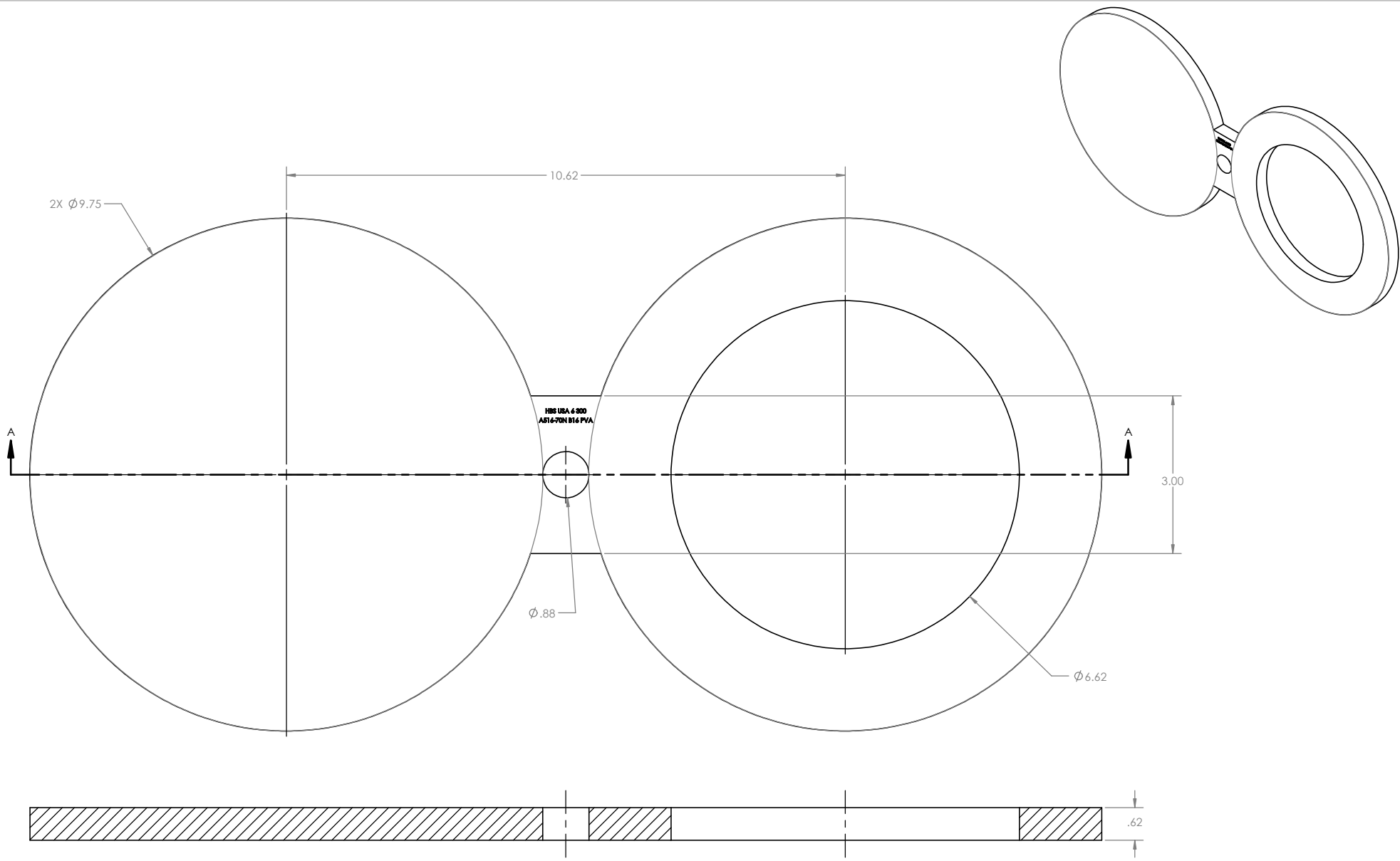
SECTION A-A
